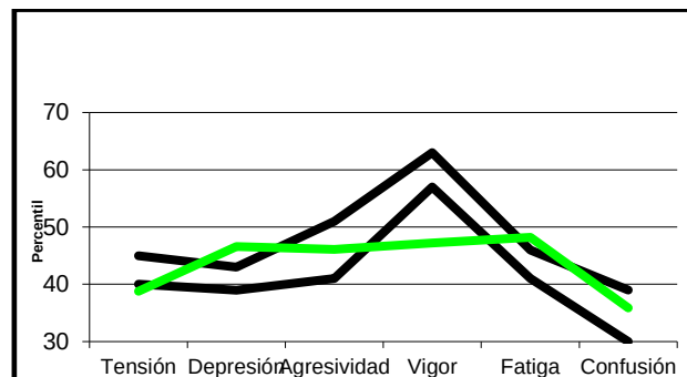
Fig.5: Resultat Test POMS inicial
